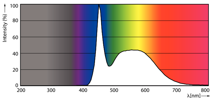
LEDtube_18W_G13_2100lm_865
