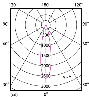
LEDspots GMGC 1 6,5W MR16 GU5,3 940 24D-LDD
