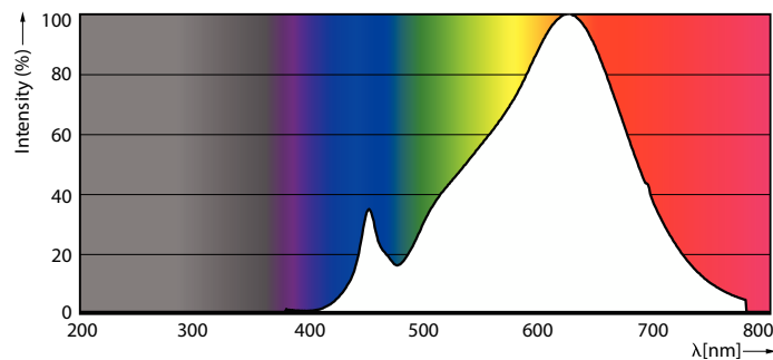
LEDspots GMGC 1 6,5W MR16 GU5,3 927 60D-POC
