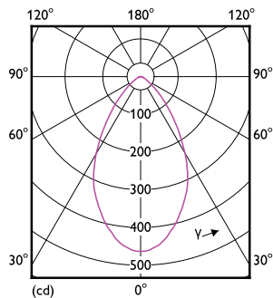
LEDspots GMGC 1 6,5W MR16 GU5,3 927 60D-LDD
